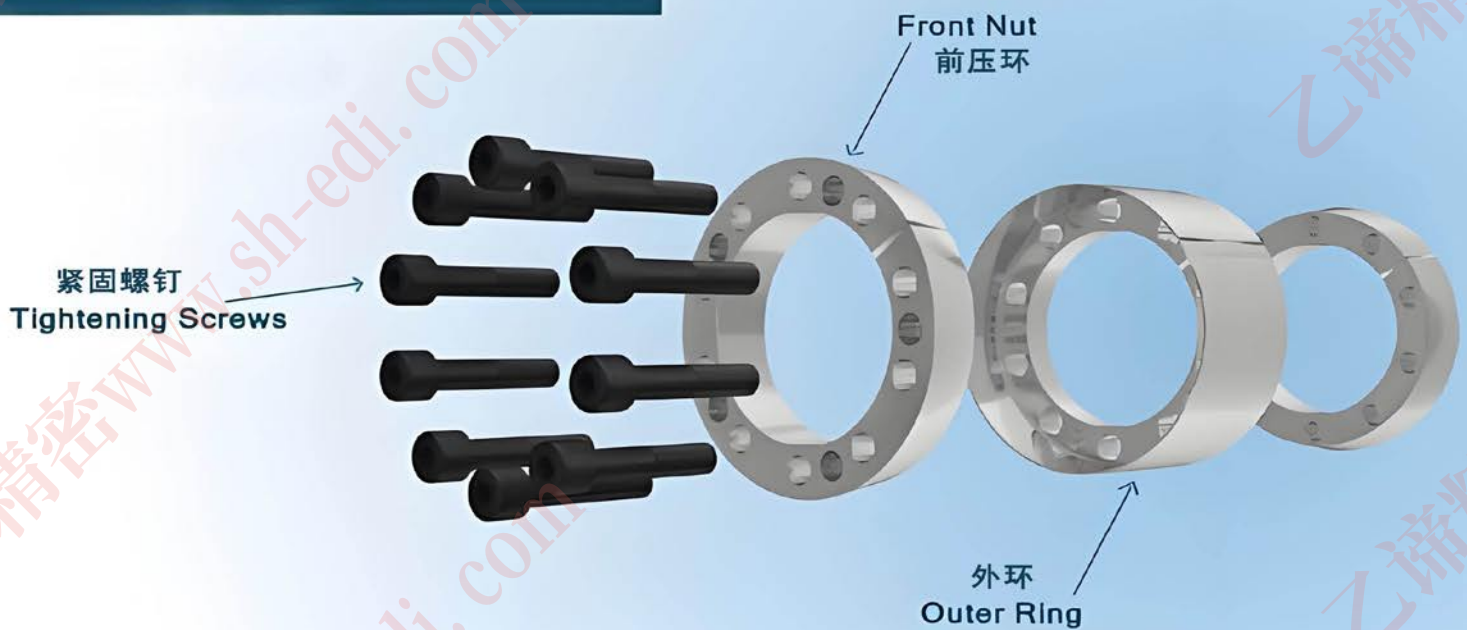
胀紧套 结构分解示意图
