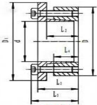
Z6 型胀紧套
